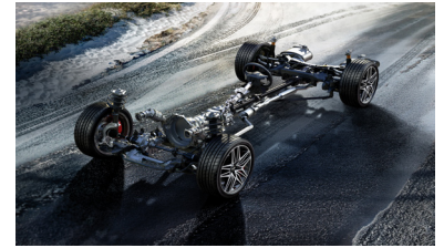
Automata összkerék-hajtás
